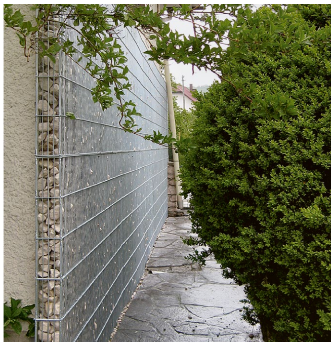
Fassadenkörbe
